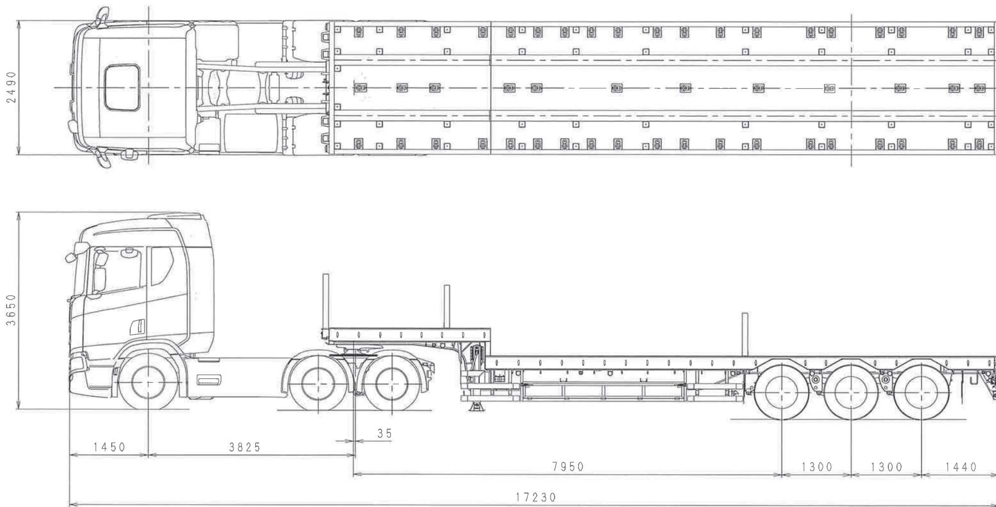
スカニア 型式不明トラクタ 東 邦 TE50J2C3S型セミトレーラ
